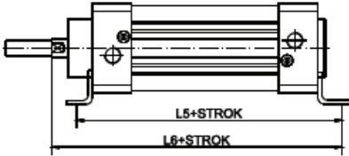
AYAK BAĞLANTI / FOOT MOUNTING
