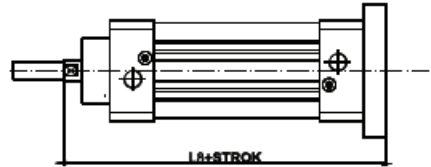
ARKA FLANŞ BAĞLANTI / REAR FLANGE MOUNTING
