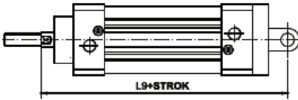
EKLEM BAĞLANTI / SWIVEL FLANGE
