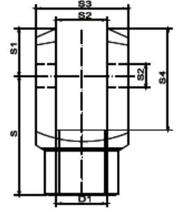
ÇB:ÇATAL BAĞLANTI / ROD CLEVIS
