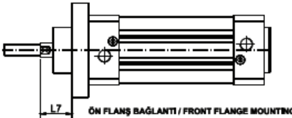
ÖN FLANŞ BAĞLANTI / FRONT FLANGE MOUNTING
