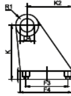
YB:YER BAĞLANTI / CLEVIS FOOT MOUNTING
