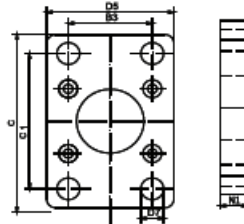
FB:FLANŞ BAĞLANTI / FLANGE MOUNTING
